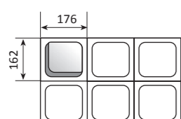
GN 1/6 176 X 162
