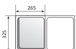
GN 1/2 325 X 265
