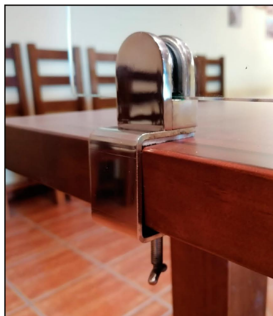
● Detalle anclaje
