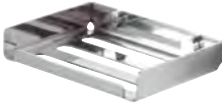
041700 Esponjara chapa inox. AISI 304 espesor 1,5 mm. brillo Shower basket polished stainless steel AISI 304
