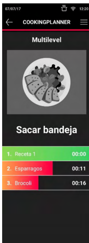
Figura 24. Opción Multilevel
