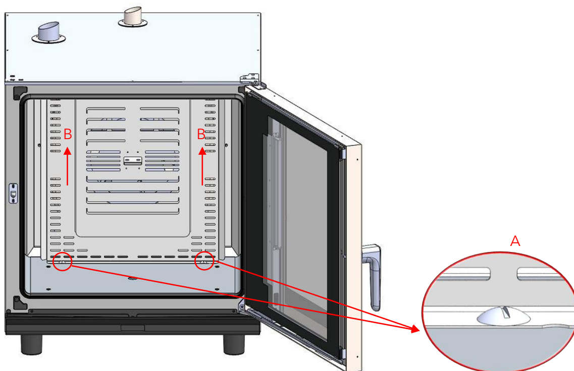
Figura 55. Sistema de fijación de la protección del ventilador e intercambiador
