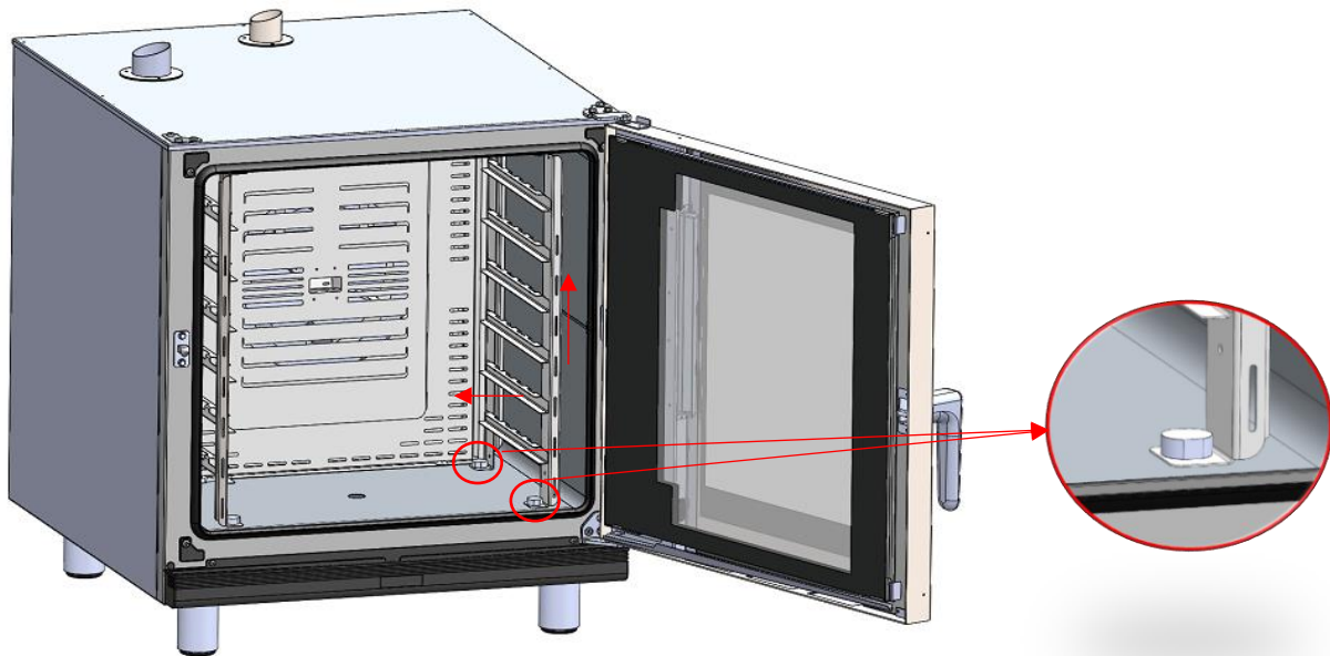
Figura 56. Detalle proceso de retirar el cuerpo de guías
