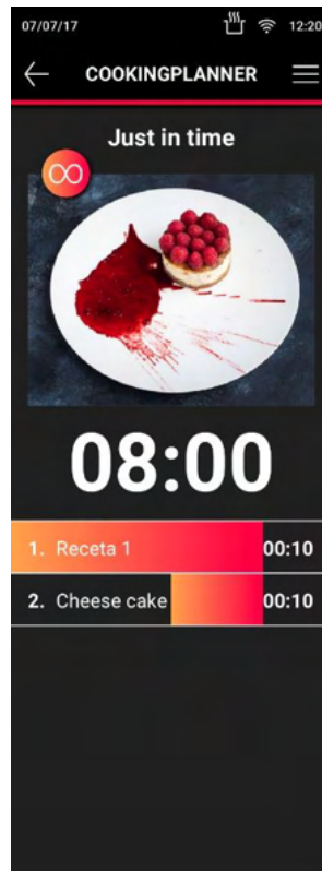
Figura 25. Opción JustInTime
