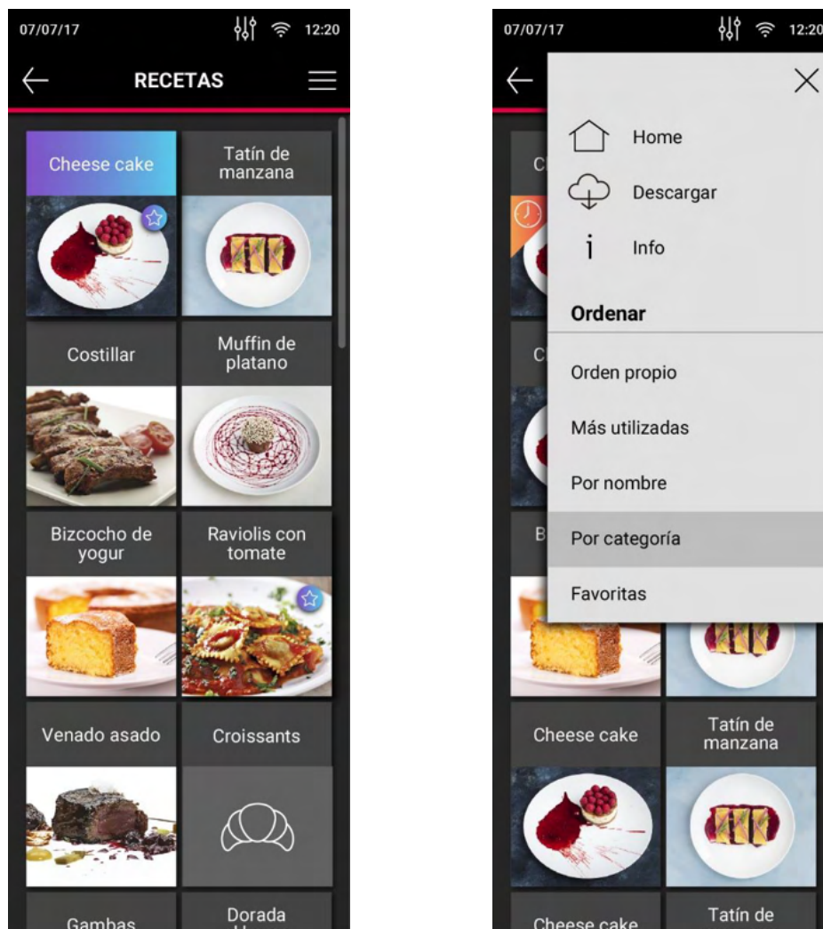
Figura 37. Opción recetas
