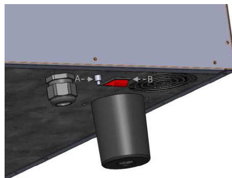
Figura 9. Termostato de seguridad (A) e interruptor de servicio (B) para BAKERSHOP 4,6,10 (600x400)
