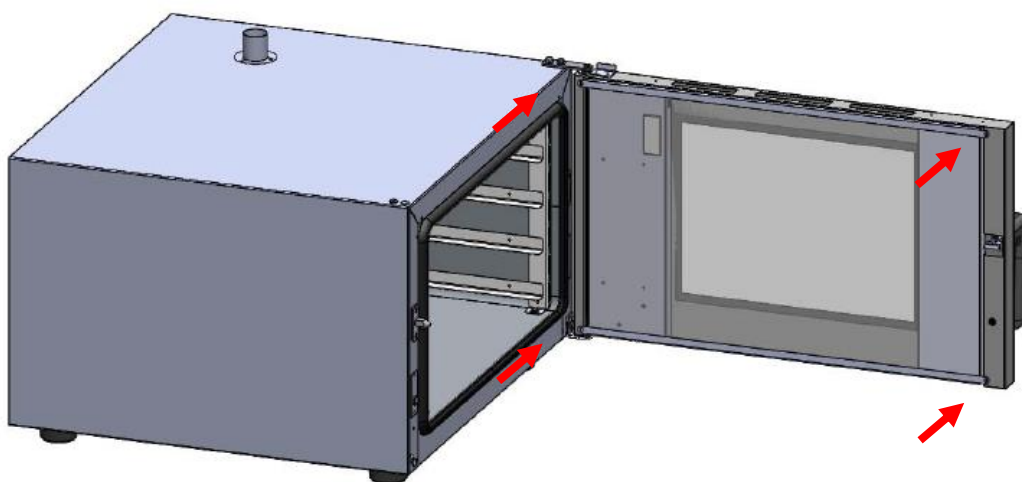
Figura 44. Tornillos de sujeción del cristal interior
