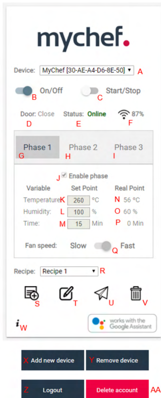
Figura 28. Detalle del panel de control
