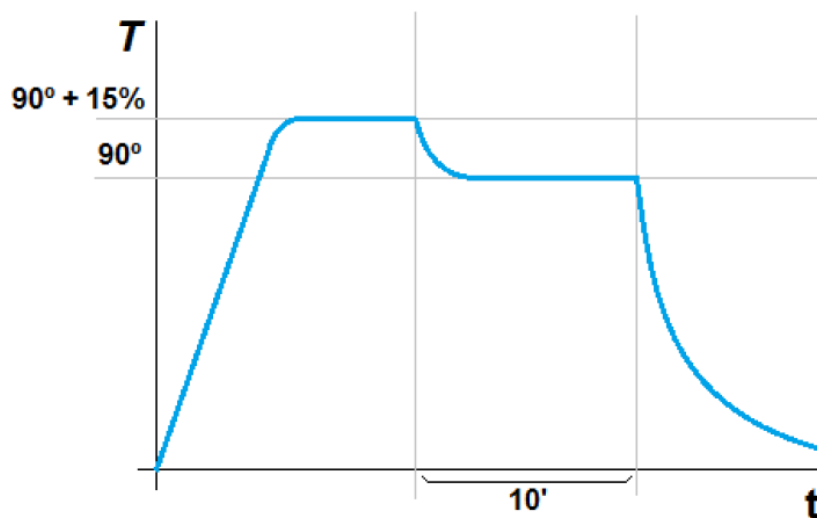
Figura 13. Temperatura horno
