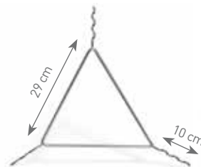
Triángulo equilátero Equilateral triangle Triangle équilatéral Gleichseitiges Dreieck
